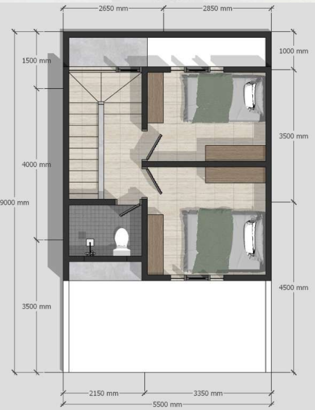
Lantai 2
