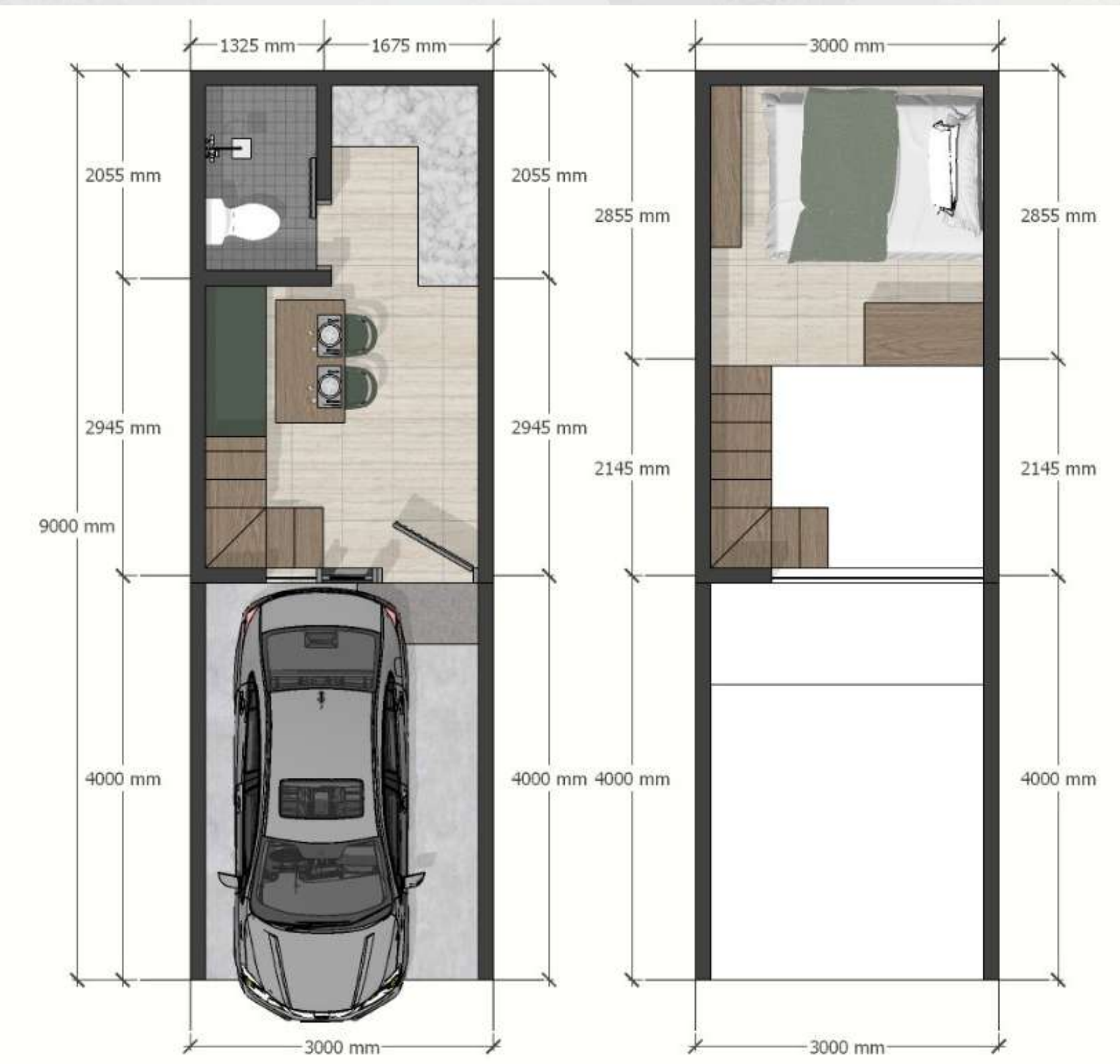
Lantai 1 Tinggi plafon: 2,5 m
