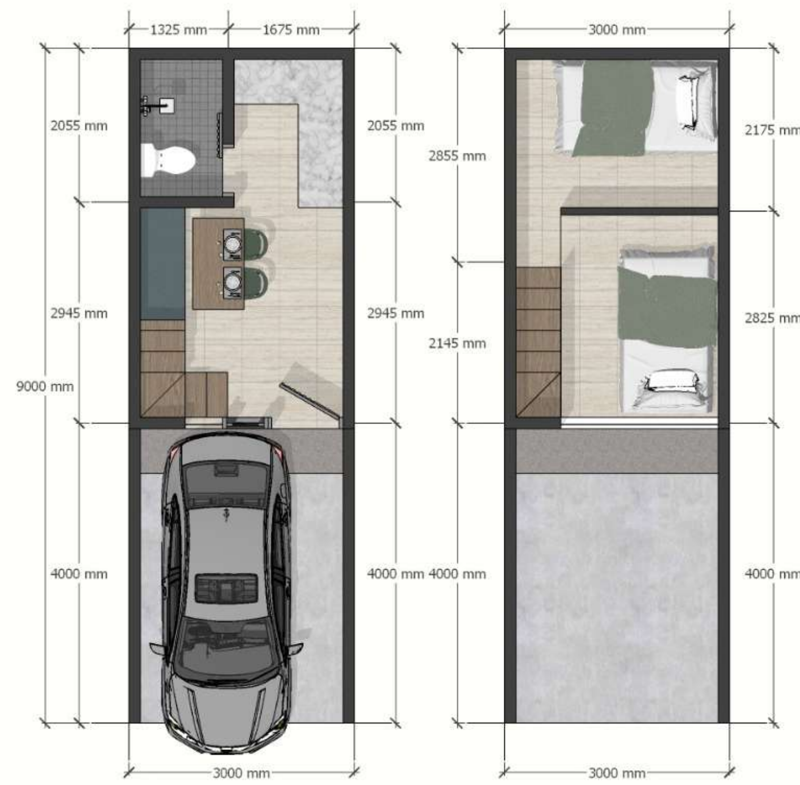
Lantai 1 Tinggi plafon: 2,5 m
